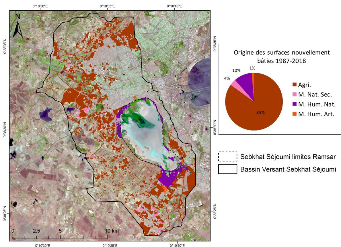
Figure 19 : Etalement des zones de bâtis entre 1987 et 2018 au sein du BV de Sebkhât Séjoumi.
