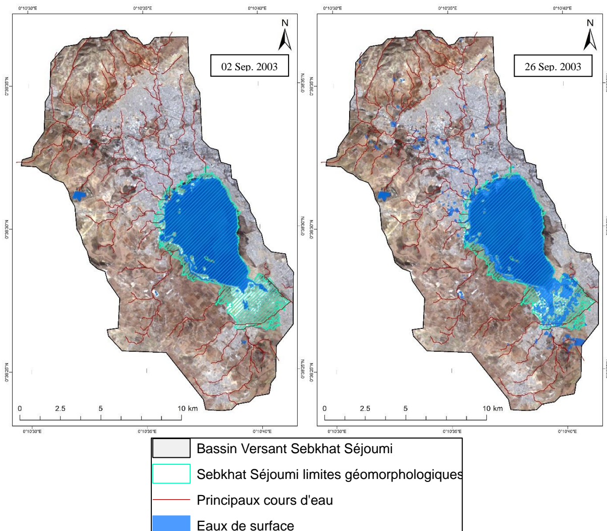
Figure 28 : Etendues des superficies en eau libre dans le BV de Sebkhât Séjoui, capturées avant et après les épisodes de pluie centennale de septembre 2003 (image de fond Landsat-TM 2003-09-02).
