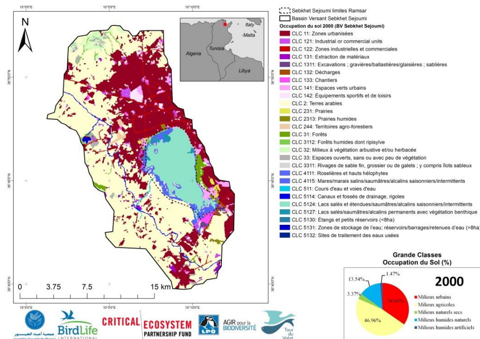
Figure 15 : Carte d'occupation du sol 2000 à l'échelle du BV de Sebkhat Séjoumi.
