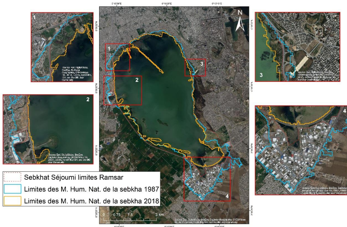
Figure 27 : Recul des berges de Sebkhata Séjoumi entre 1987 et 2018, suite aux remblaiements et aux constructions successifs.
