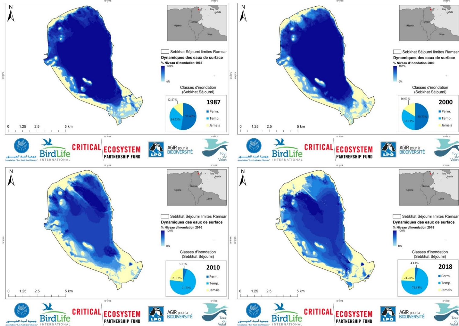
Figure 6 : Cartes des régimes des eaux de surface au sein des limites Ramsar de Sebkhât Séjoumi pour les hydropériodes annuelles 1987, 2000, 2010 et 2018.
