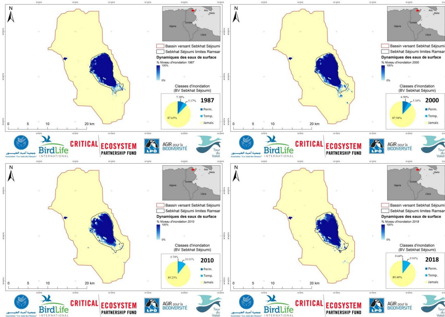
Figure 4 : Cartes des régimes des eaux de surface à l'échelle du BV de Sebkhât Séjoumi pour les hydropériodes annuelles 1987, 2000, 2010 et 2018.
