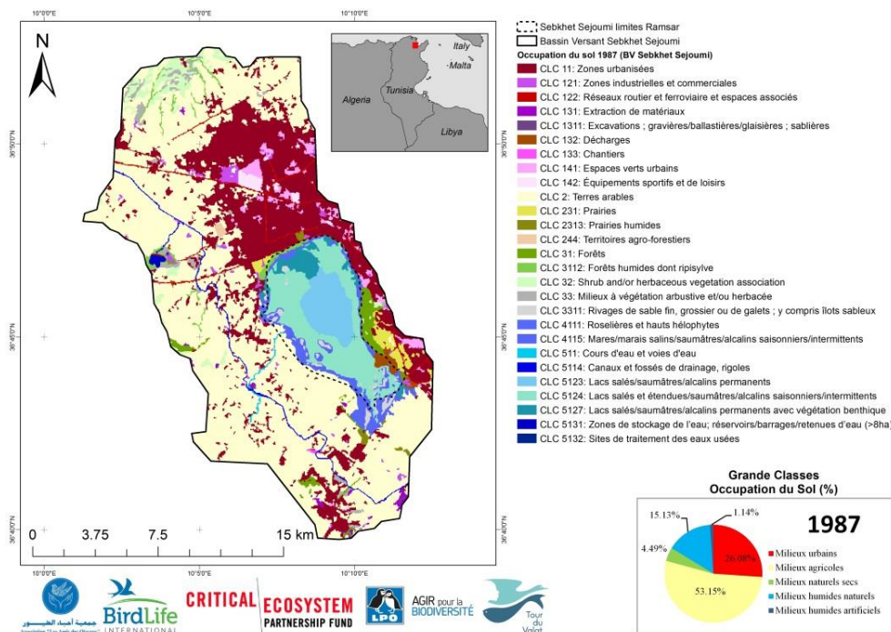
Figure 14 : Carte d'occupation du sol 1987 à l'échelle du BV de Sebkhat Séjoumi.
