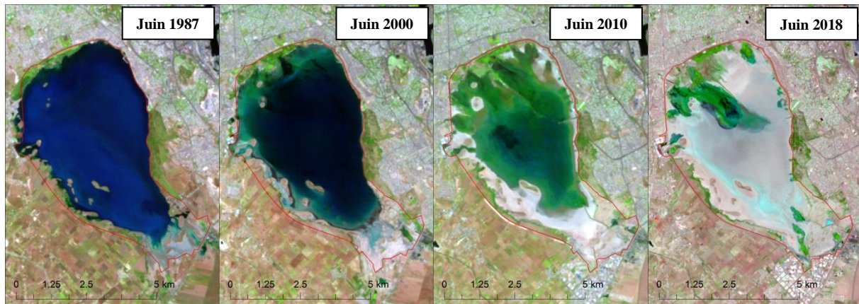
Figure 12 : Images satellites de Sebkhât Séjoumi à la même période annuelle (juin) en 1987, 2000, 2010 et 2018. A noter son assèchement progressif et de plus en plus long et précoce durant la saison estivale à cause, notamment, du système de pompage automatique mis en place à partir de 2004 (R/G/B : MIR/PIR/R).
