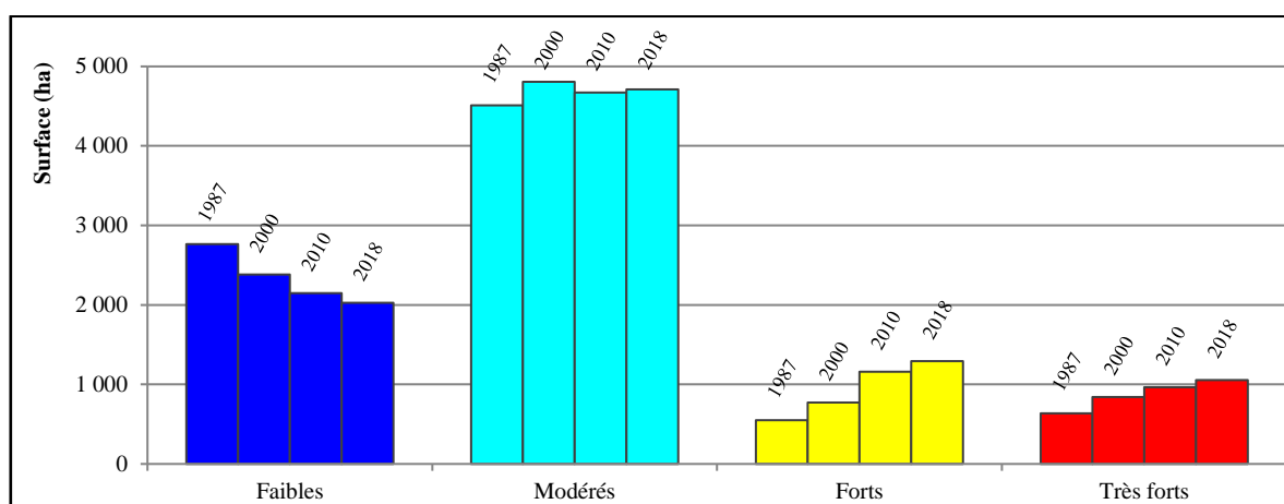
Figure 26 : Evolution des enjeux socio-économiques (représentés ici en superficies) face aux risques de crue et de débordement des eaux de surface au sein du territoire du BV de Sebkhât Séjoumi entre 1987 et 2018.
