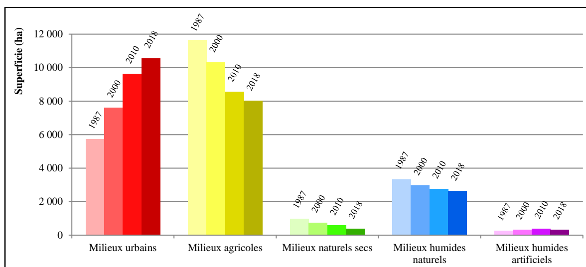
Figure 18 : Evolution des grandes classes d'occupation du sol au sein du BV de Sebkhath Séjoumi, entre les hydropériodes annuelles 1987, 2000, 2010 et 2018.
