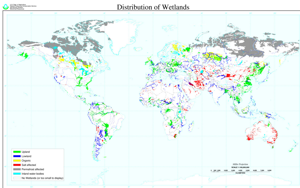
Figure I. Répartition des zones humides à l'échelle mondiale
